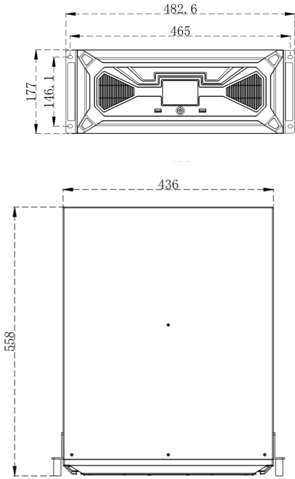
设备尺寸图
