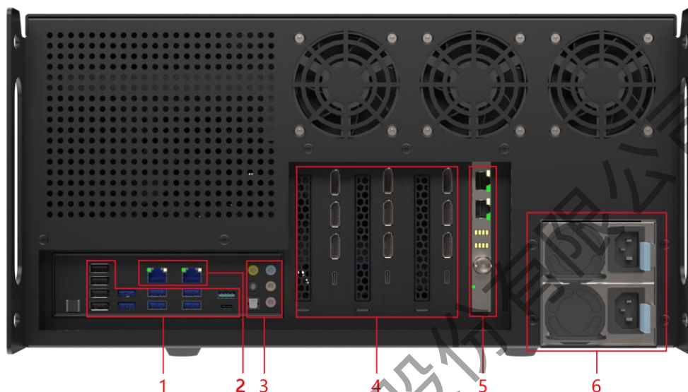
设备背面图
