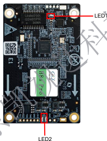
前面板外观
