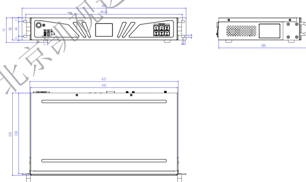
设备尺寸图
