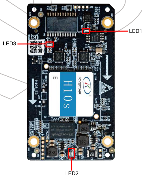
前面板外观
