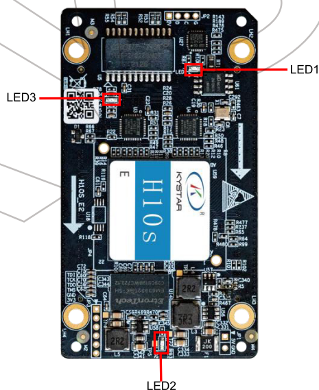
前面板外观
