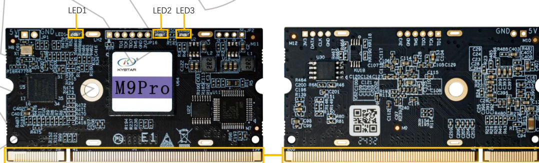
金手指接口
