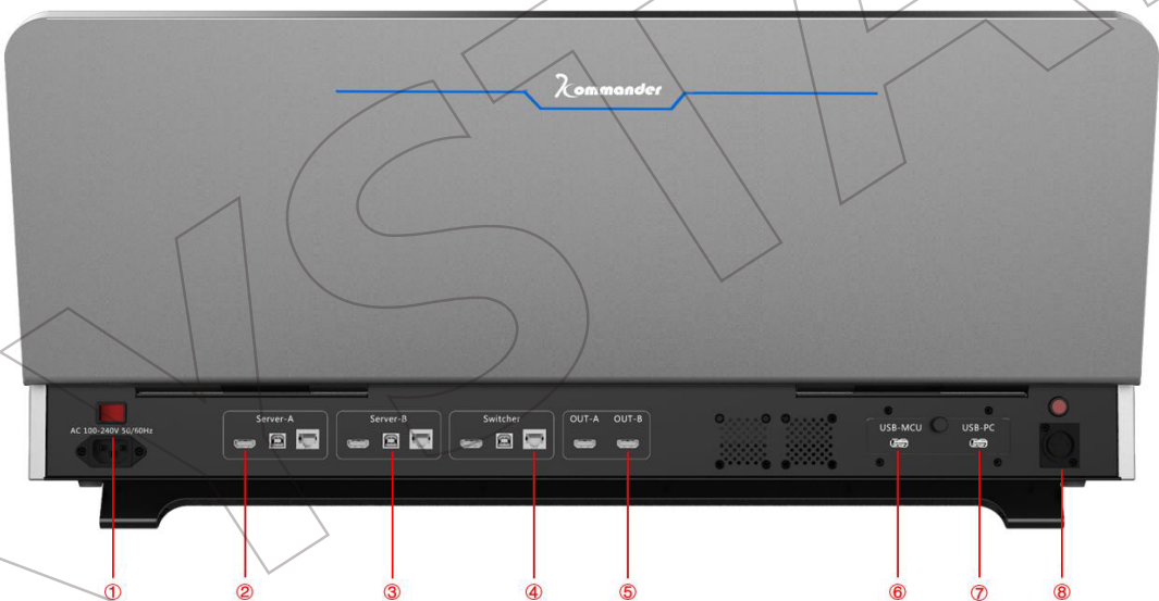
设备背面图
